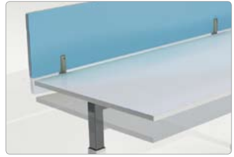
Altura ajustável de 62 a 86 cm. Height range from 62 to 86 cm.
